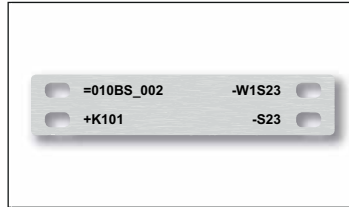
Kabelschild 12 x 60 mm, mit Bohrungen, Maßstab 2:1
